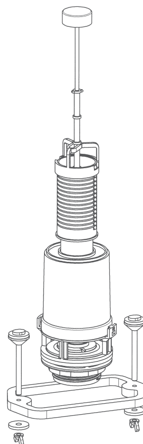
Adapté aux dimensions du réservoir ASPIRAMBO PORCHER
