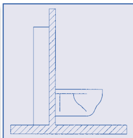
En gaine technique (épaisseur maxi du mur 100 mm)
