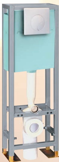
Bâti-chasse VERSO BCS 350 complet ( sortie Ø 100 mm )
