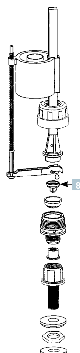
BAS 26EL
