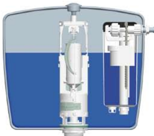
ROBINET FLOTTEUR EN POSITION FERMÉE
