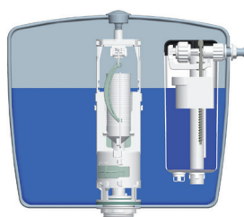
ROBINET FLOTTEUR EN POSITION FERMÉE
