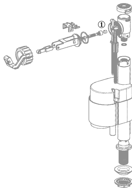
① Clapet
