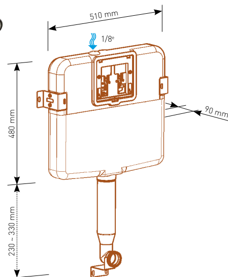
Fixation arrière
