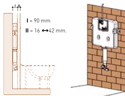
Fixation arrière
