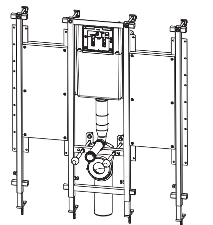
MONTAGE DU PANNEAU EN POSITION BASSE
