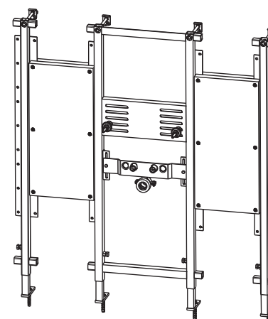
MONTAGE DU PANNEAU EN POSITION BASSE
