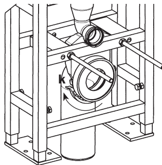
Sortie coudée
