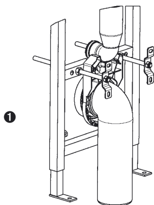
Sortie coudée
